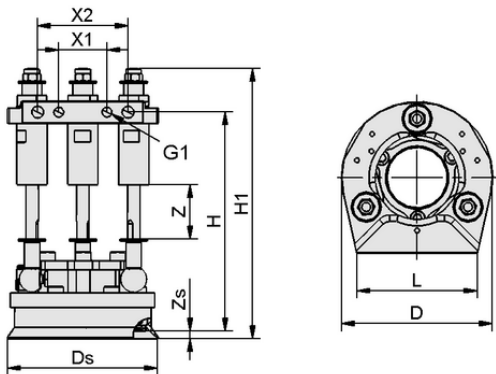
设计参数 DBD 100x189 80 M42
