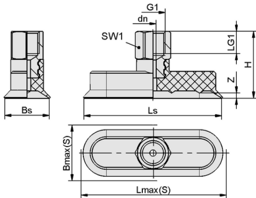
设计参数 SGON 60x20 NBR-55 G1/4-IG
