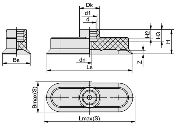
设计参数 SGO 90x30 NBR-70 N023
