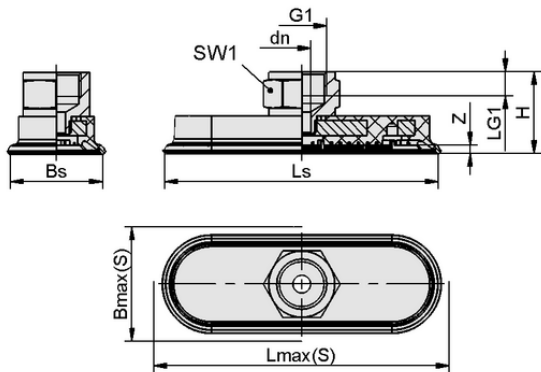
设计参数 SAOF 60x23 NBR-45 G1/4-IG
