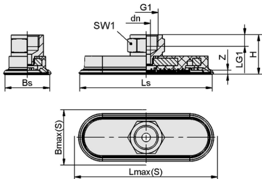
设计参数 SAOF 60x23 NBR-45 G3/8-IG
