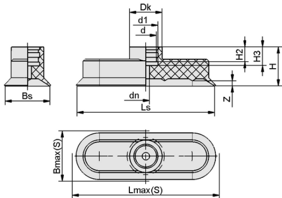
设计参数 SGO 24x8 NBR-CO-55 N022
