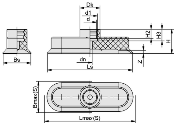
设计参数 SGO 75x25 SI-HD-65 N023
