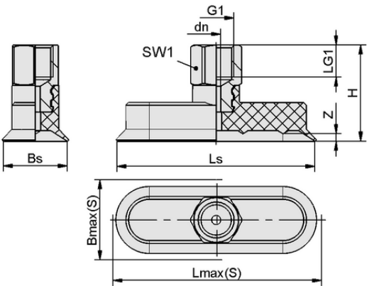
设计参数 SGON 15x5 SI-HD-65 M5-IG
