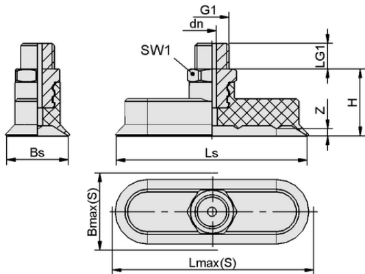
设计参数 SGON 15x5 SI-HD-65 M5-AG
