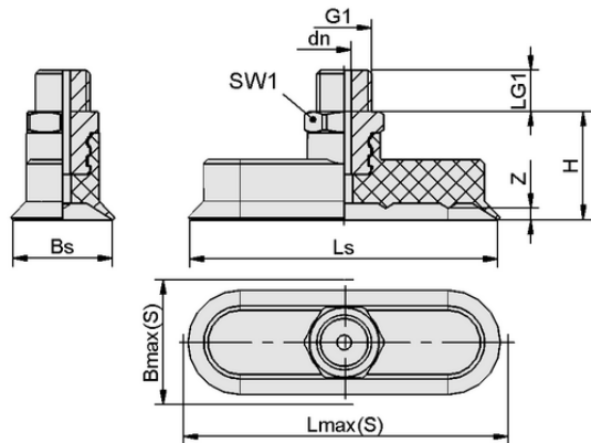
设计参数 SGON 45x15 SI-HD-65 G1/4-AG
