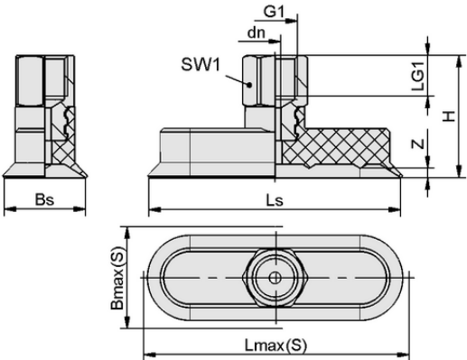
设计参数 SGON 60x20 SI-HD-65 G1/4-IG
