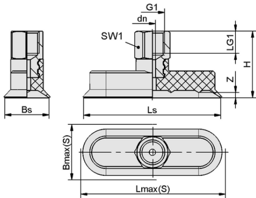
设计参数 SGON 75x25 SI-HD-65 G1/4-IG
