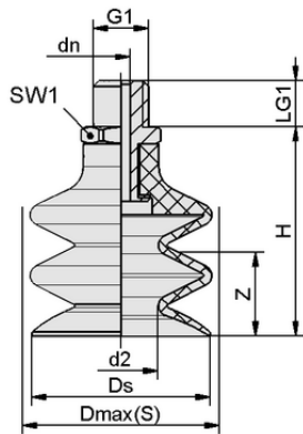
设计参数 FSG 42 NBR-55 G1/4-AG
