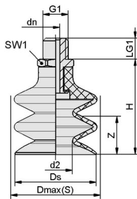
设计参数 FSG 20 SI-55 G1/8-AG
