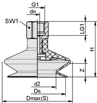
设计参数 FSGA 53 NBR-55 G1/4-IG
