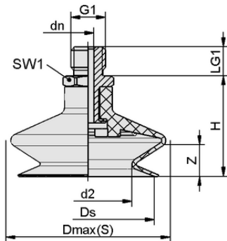
设计参数 FSGA 16 NBR-55 M5-AG
