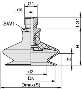
设计参数 FSGA 78 NK-45 G1/4-AG
