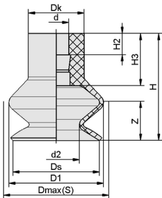
设计参数 FGA 25 NK-45 N016
