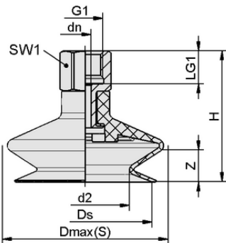
设计参数 FSGA 25 SI-55 G1/8-IG
