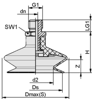
设计参数 FSGA 16 NK-45 G1/8-AG
