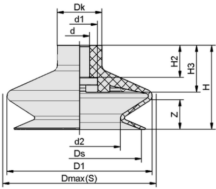
设计参数 FGA 63 SI-55 N018
