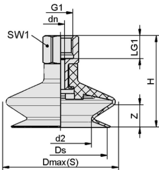
设计参数 FSGA 63 NBR-55 G1/4-IG
