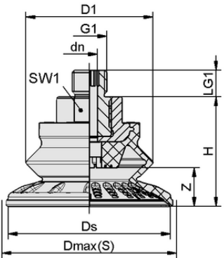
设计参数 SAB 40 NBR-60 M14x1.5-AG
