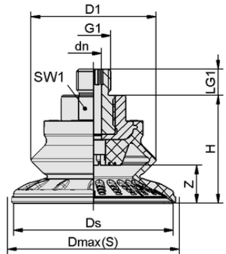
设计参数 SAB 50 NBR-60 M14x1.5-AG
