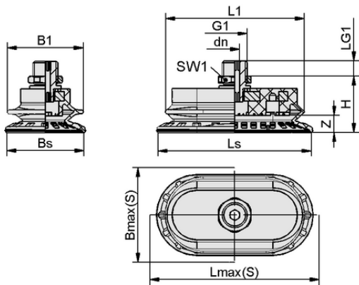
设计数据 SAOB 80x40 NBR-60 M10-AG
