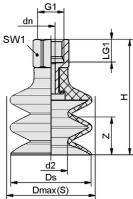
设计参数 FSG 7 HT1-60 G1/8-IG
