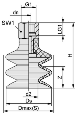
设计参数 FSG 12 HT1-60 G1/8-IG
