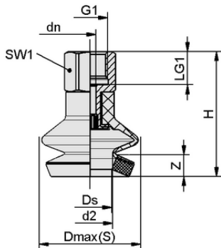
设计参数 FSGA 33 NK-45 G1/4-IG DR
