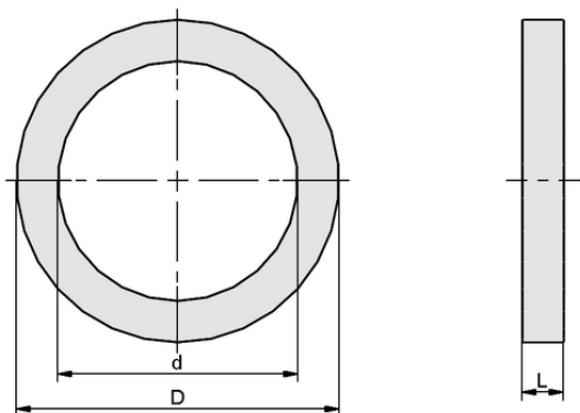
设计参数 DR 28/21x3 C03 EPDM-15 KE
