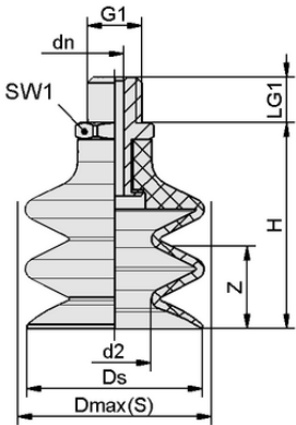
设计参数 FSG 52 NK-45 G1/4-AG
