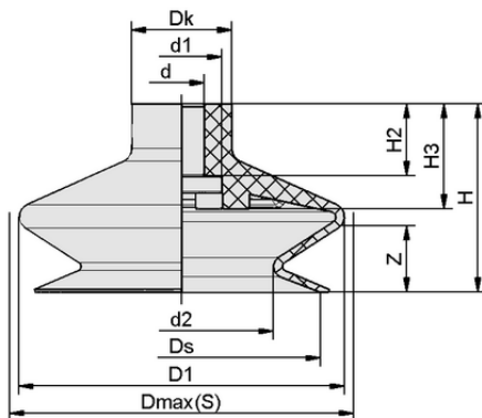
设计参数 FGA 78 HT1-60 N019
