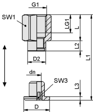
设计参数 SC 050 G1/4-IG MOD
