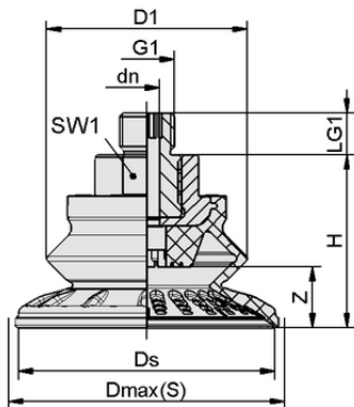
设计参数 SAB 60 HT1-60 G1/4-AG
