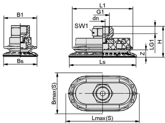
Design data SAOB 60x30 HT1-60 G3/8-IG
