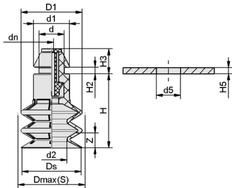
设计参数 SPB2 20 SI-40 SW100 P
