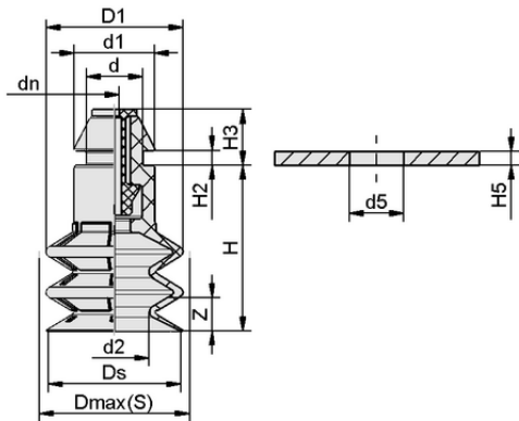
设计参数 SPB2 20 SI-40 SW150 P
