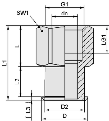
设计参数 SC 090 G1/4-IG
