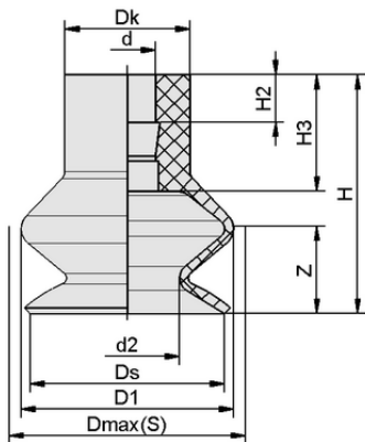
设计参数 FGA 22 SI-HD-65 N016
