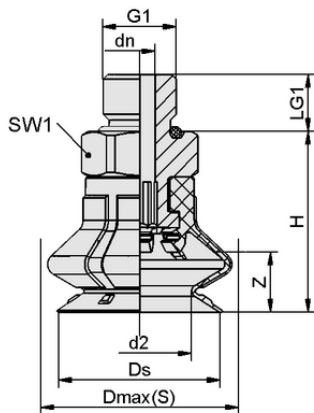
设计参数 SPB1 20 ED-65 G1/8-AG
