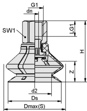
设计参数 SPB1 40 ED-65 G1/4-IG
