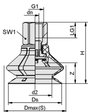
设计参数 SPB1 60 ED-65 G1/4-IG
