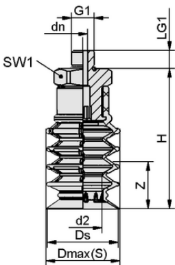
设计参数 SPB4 40 SI-55 G1/4-AG
