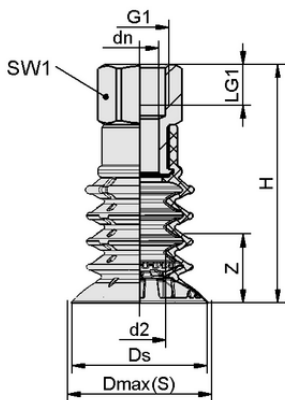
设计参数 SPB4f 30 SI-55 G3/8-IG
