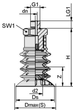
设计参数 SPB4f 40 SI-55 G3/8-AG
