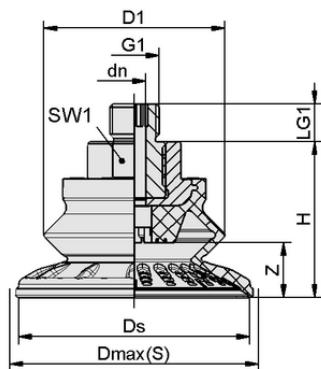
设计参数 SAB 40 NBR-60 M16-AG
