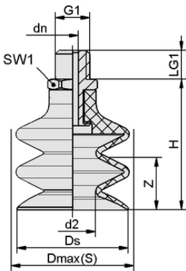
设计参数 FSG 3 SI-55 M5-AG
