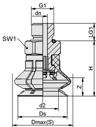
设计参数 SPB1 80 ED-65 G1/2-AG
