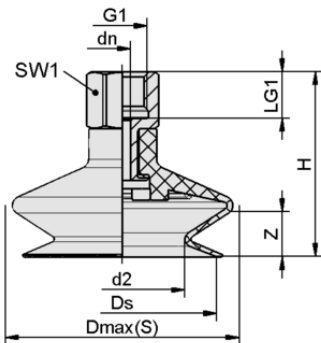
设计参数 FSGA 16 SI-MD-55 G1/8-IG
