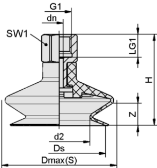
设计参数 FSGA 33 SI-MD-55 G1/4-IG
