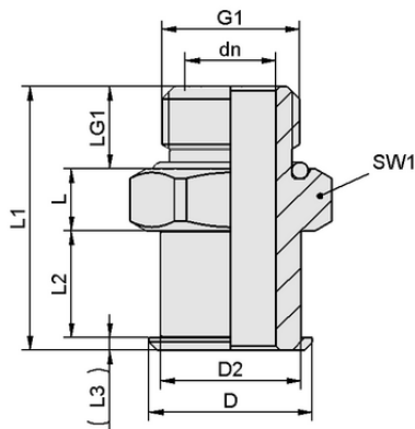
设计参数 SC 010 M3-AG
